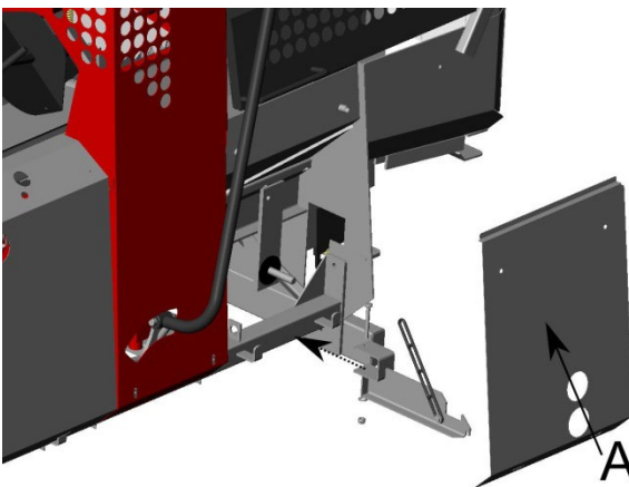
Bild 6. Låsjärn Power 70
