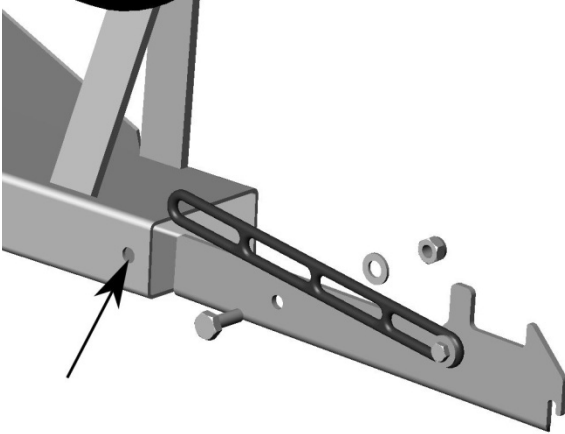
Bild 4. Låsjärn KS 35
