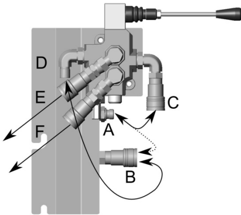
Bild 9. Montering av hydrauliken på KS 35 och Power 70
