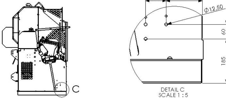
Bild 2. Borrningsanvisningar
