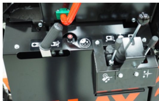
Modely Pro a Pro+: Všechny ovládací páky jsou seskupeny na jednom místě, čímž umožňují snadnou obsluhu.
