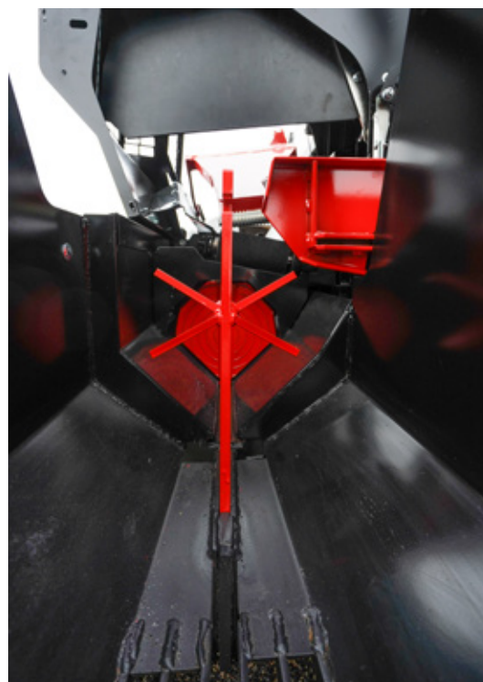
Výměna štípacího klínu je rychlá a snadná.
