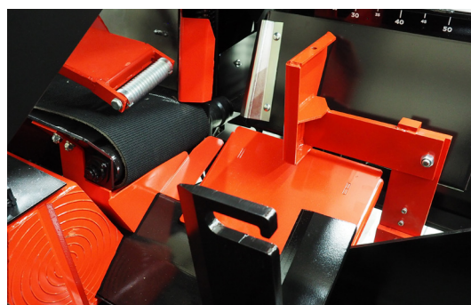
Ett hydrauliskt tippbord styr vedklabbarna rakt in i klyvrännan.
