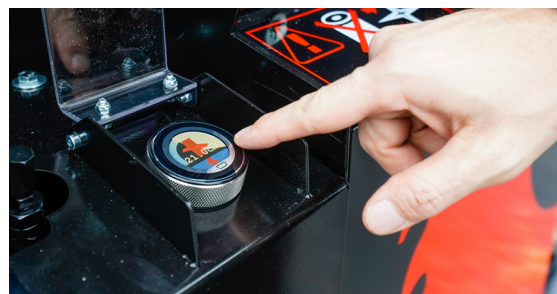
Med X-Aims intelligens får användaren även data om arbetsproduktiviteten i realtid: pekskärmen skiljer mellan bearbetade vedkubbar, användningstimmar, antal cykler och sågkvadrater.
